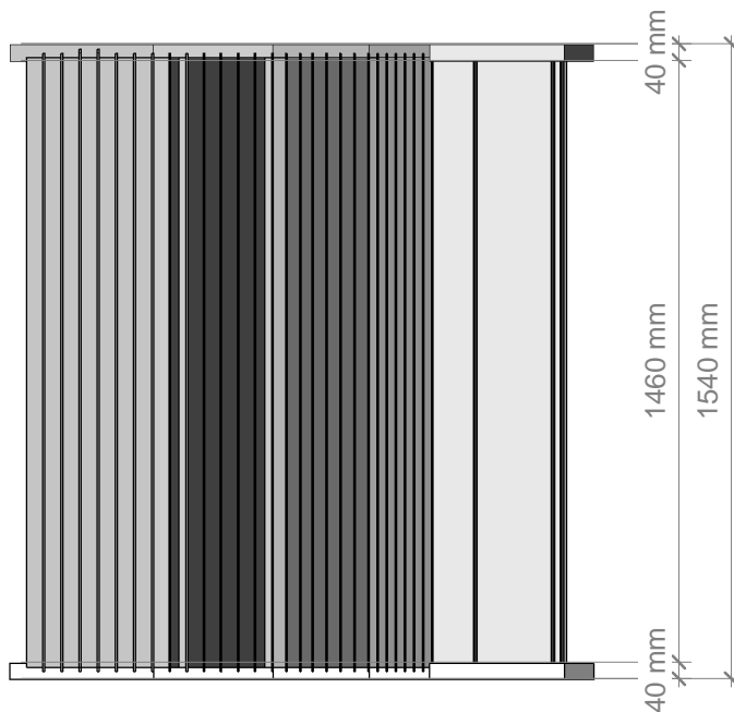
1 Elevation 1 : 20
