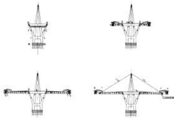
Viadotto sul Polcevera. Costruzione senza centine
