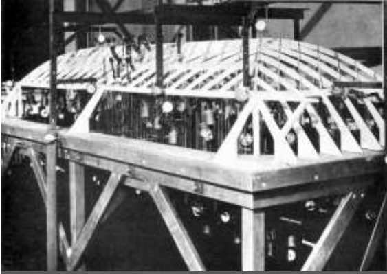
Nervi e Danusso. Modello di aviorimessa in cellulosoide, prima serie, 1935
