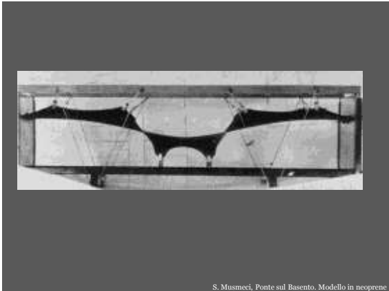
S. Musmeci, Ponte sul Basento, Modello in neoprene
