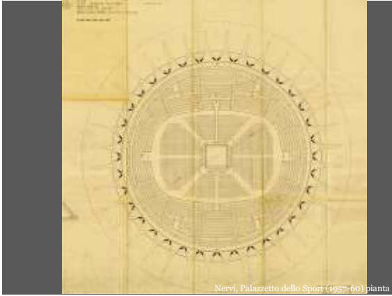
Nervi, Palazzetto dello Sport (1957-60) pianta
