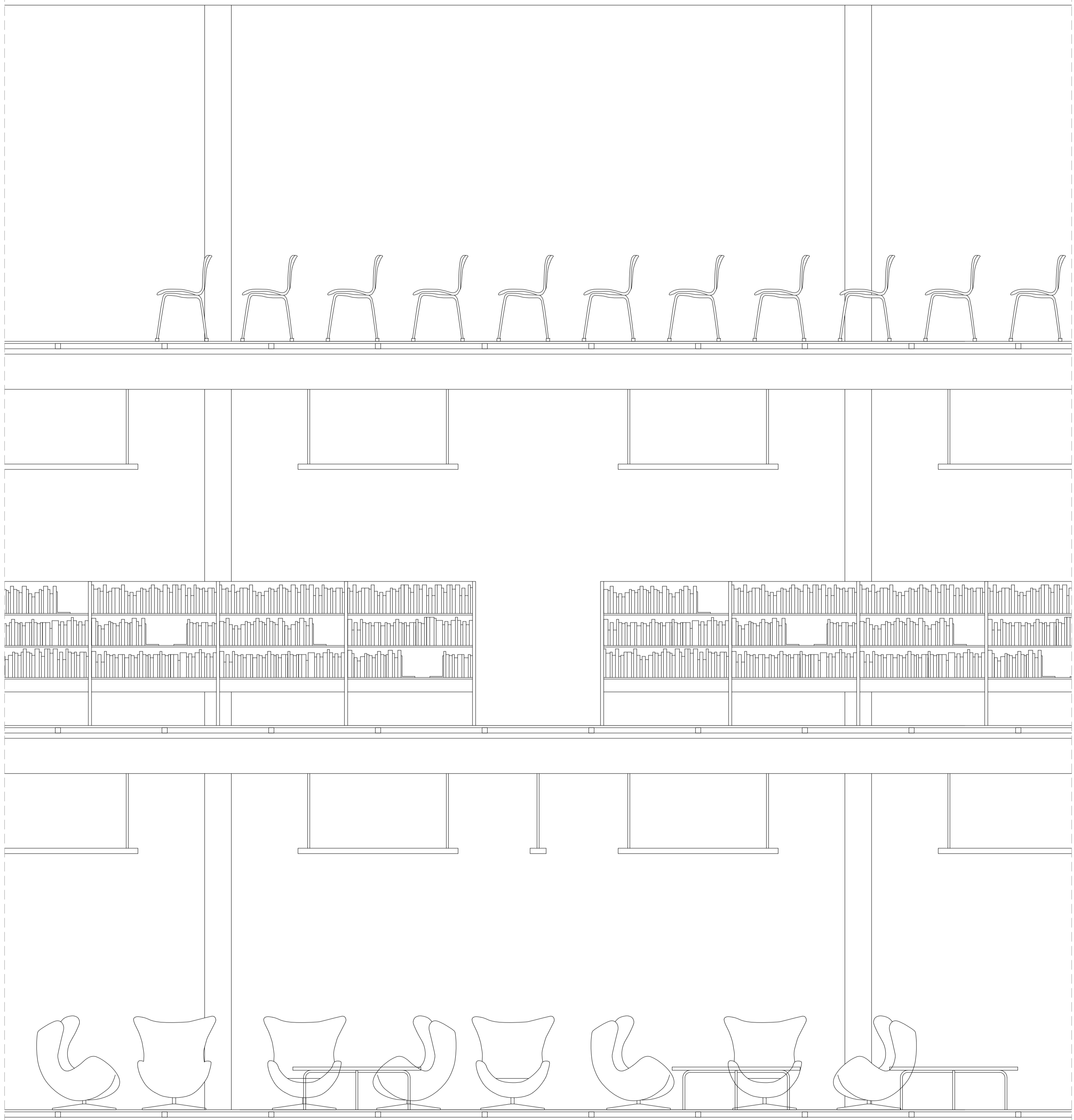
sezione C
