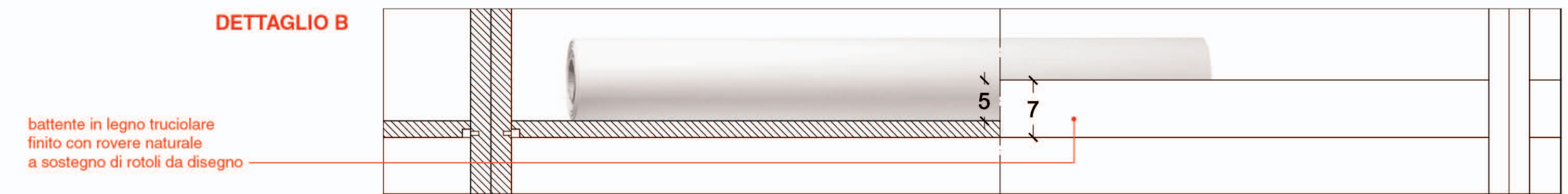
SEZIONE / PROSPETTO scala 1:5
