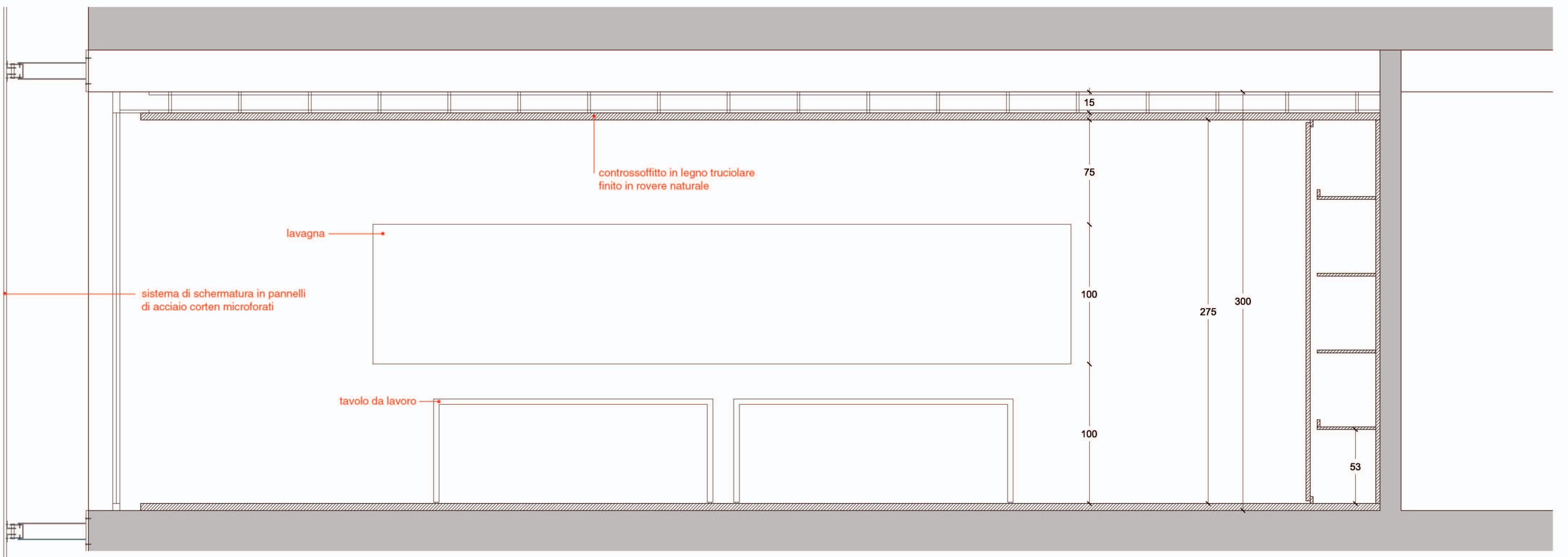
SEZIONE AA' scala 1:20
