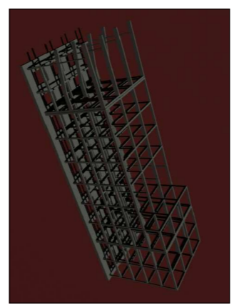
STRUTTURA A TELAMO IN CEMENTO ARMATO VISTA 1
