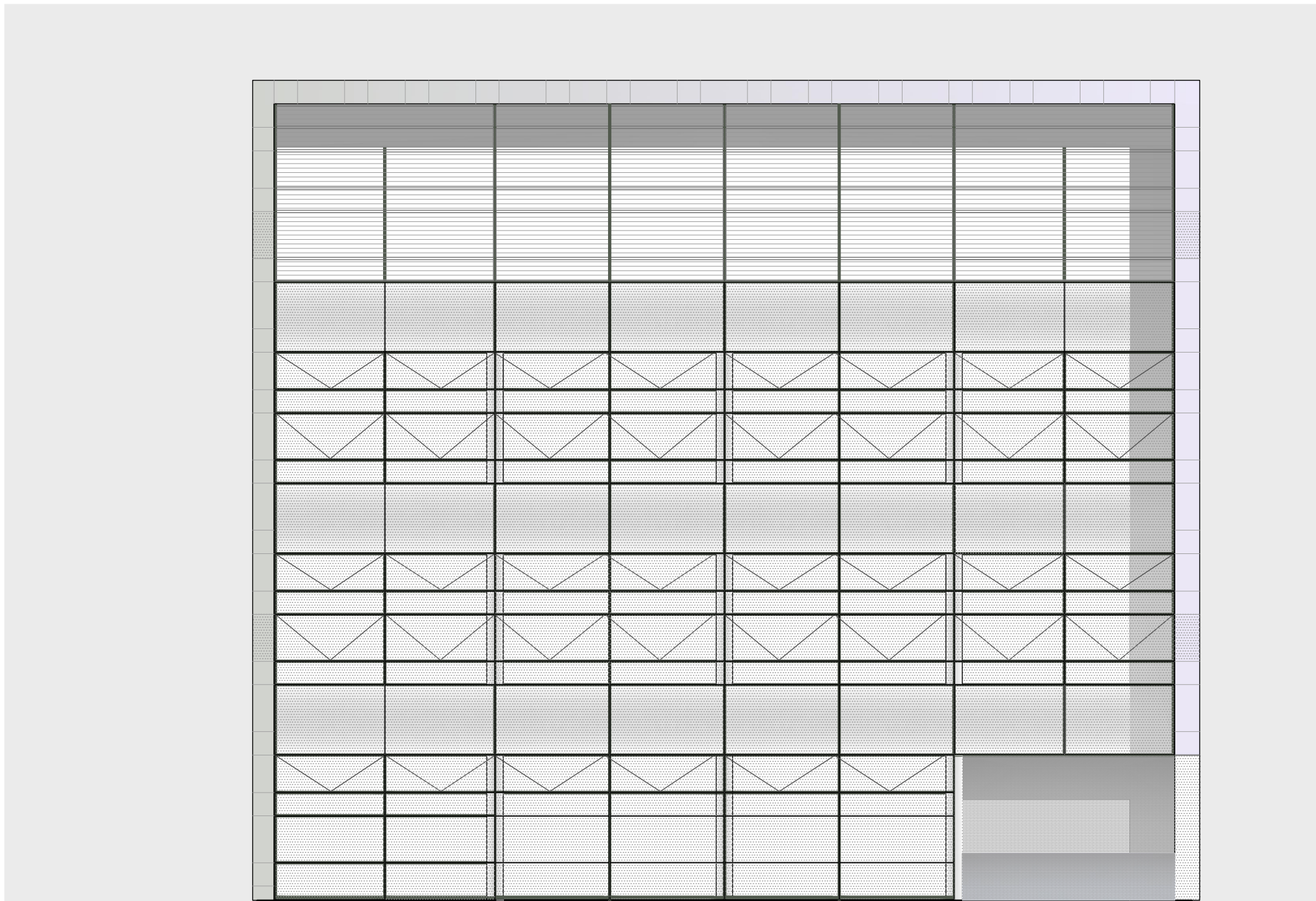
Prospetto Nord-Ovest su Via Aldo Manuzio Scala 1:100
