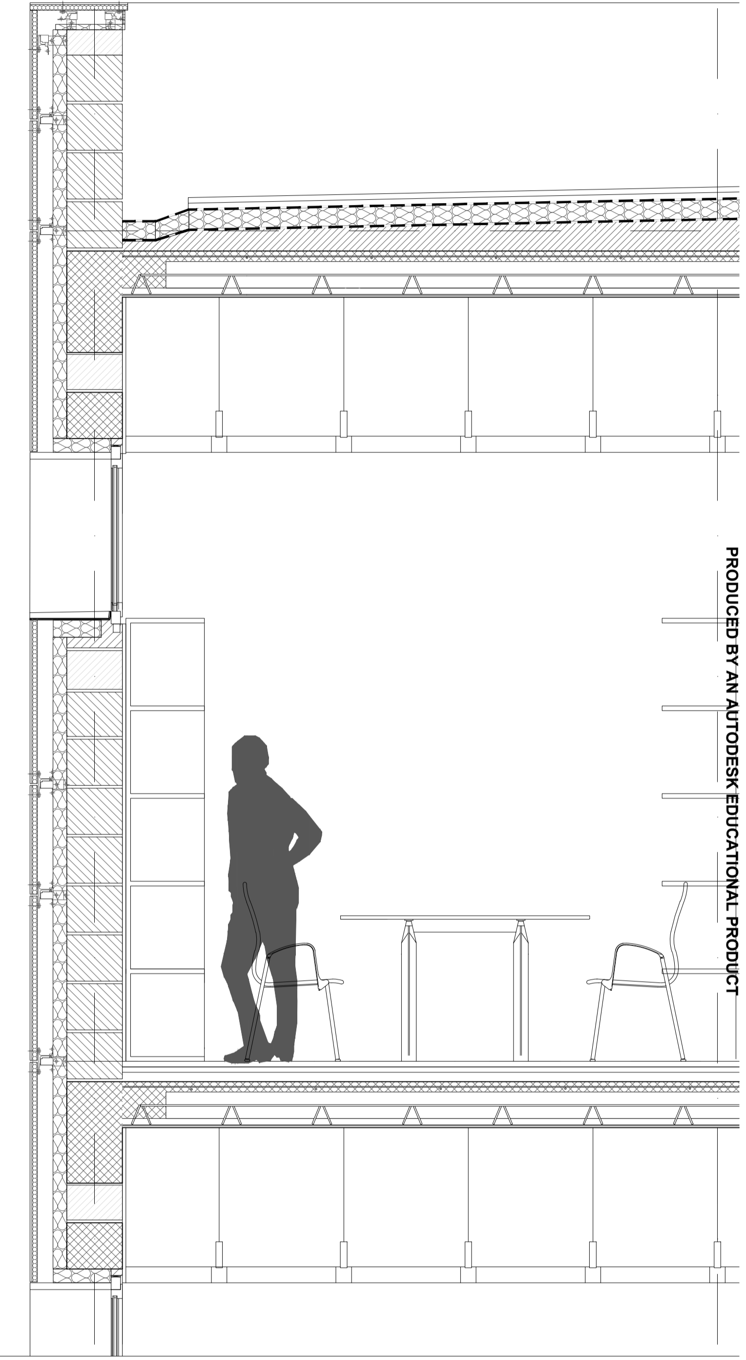
Dett 1 scala 1:20
