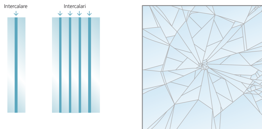
Tipo di frammentazione di un vetro stratificato.
