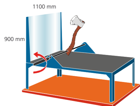
Prova dell'ascia EN 356
