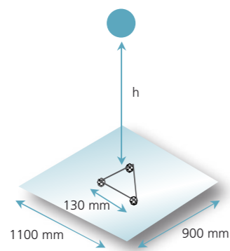
Prova della palla d'acciaio EN 356
