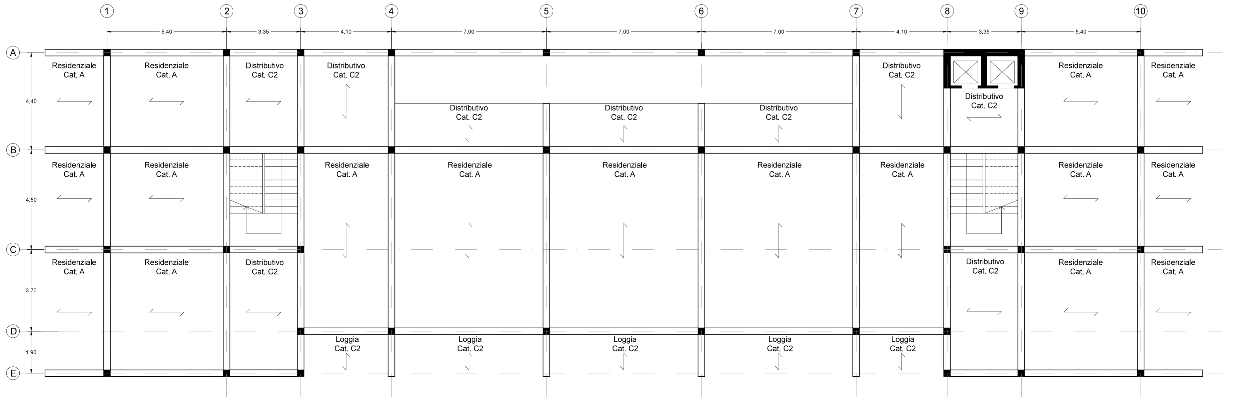
Pianta strutturale piano tipo residenziale
