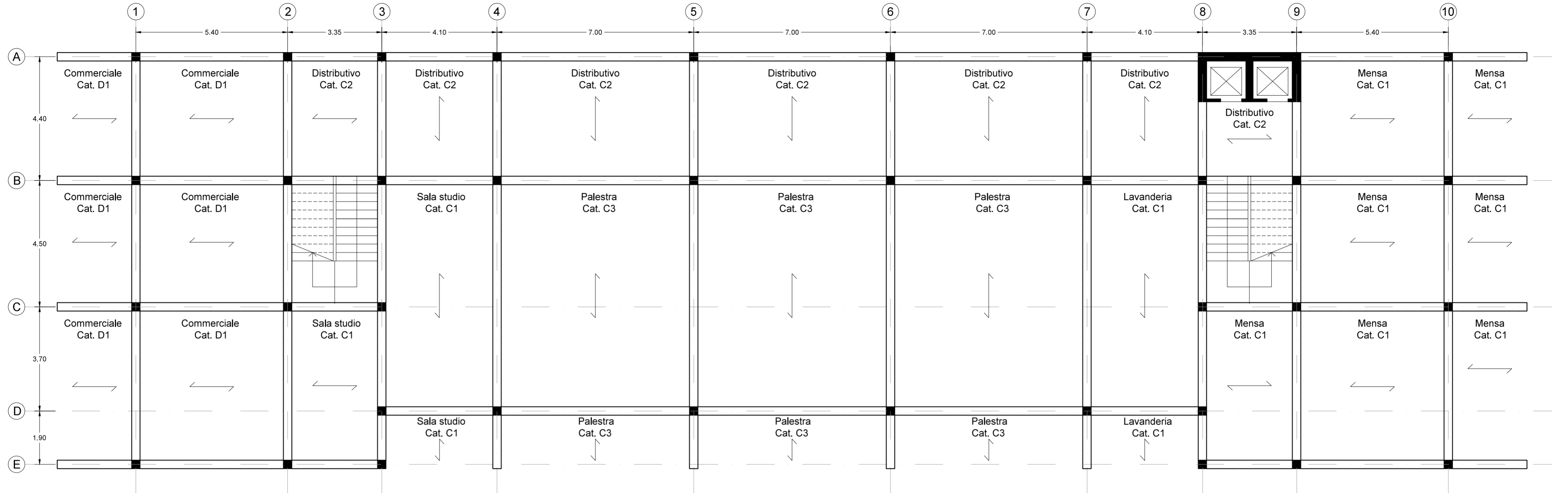
Pianta strutturale piano terra
