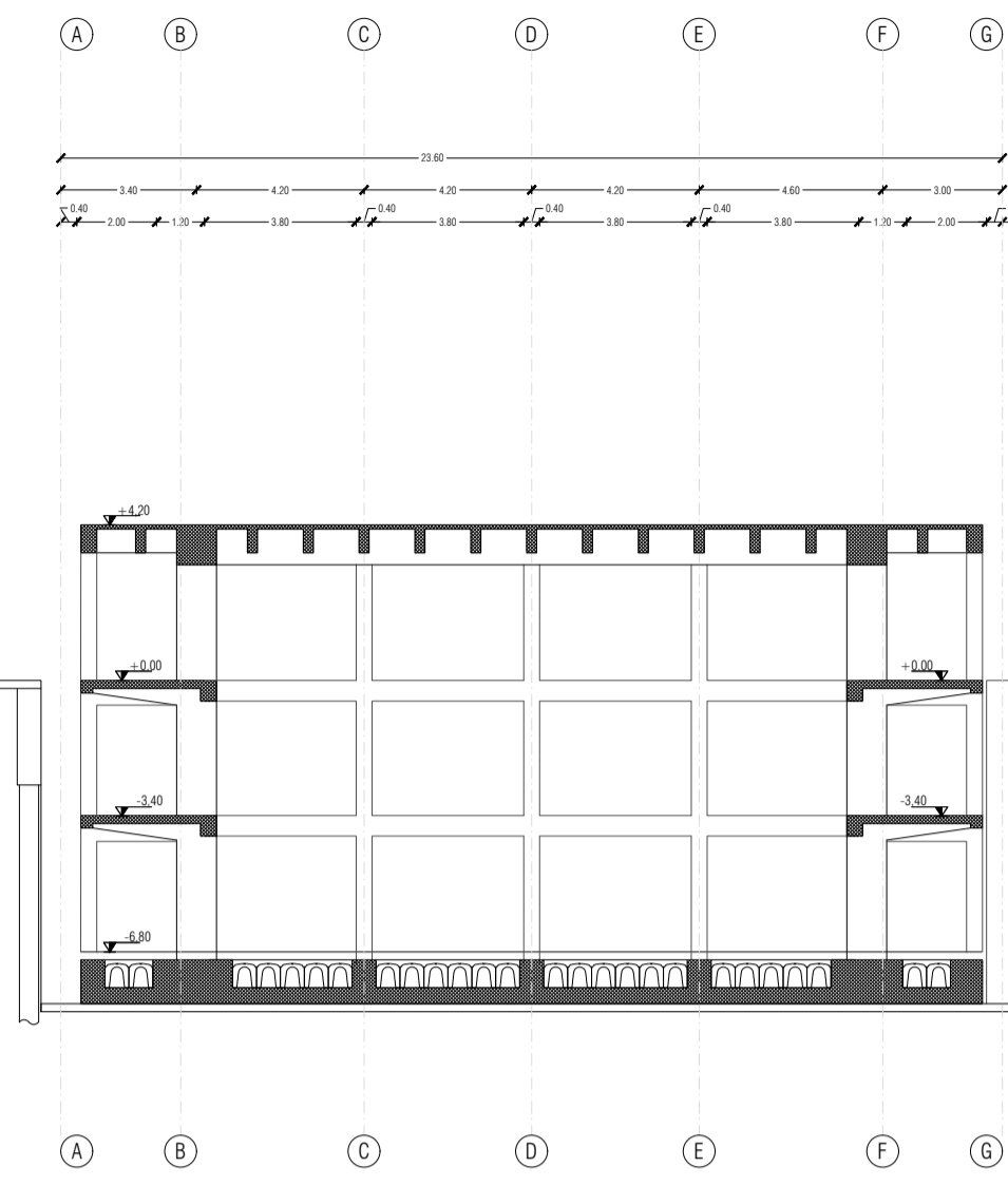
SEZIONE DD'
